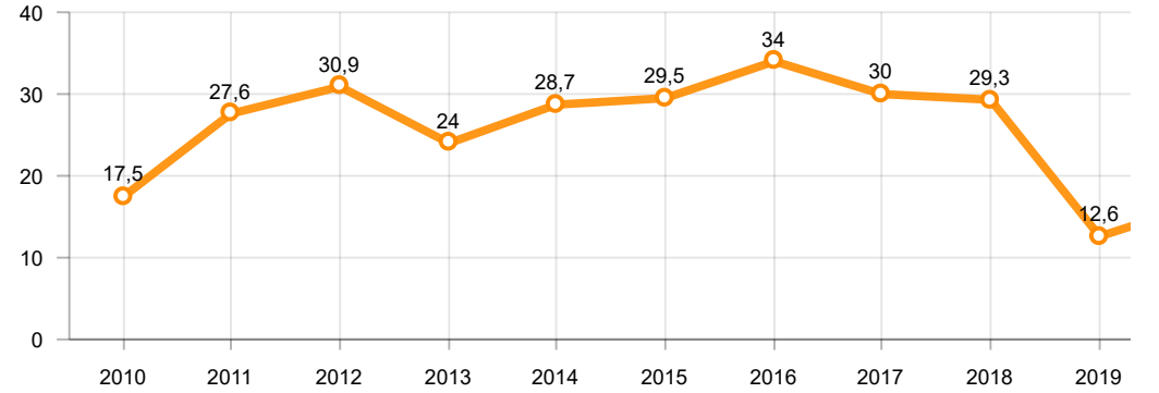
Traktör Üretimi (x1000)(OCAK - TEMMUZ) F. Tractor Production (x1000)(January - July)
